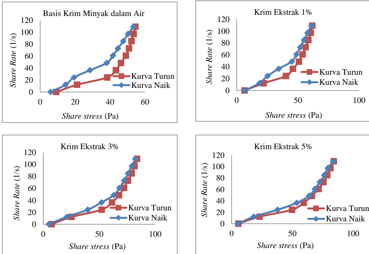
Gambar 3. Grafik rheogram hubungan antara Shearing rate (SS) vs Shearing Stress krim ekstrak buah pepaya. Berdasarkan grafi ini keempat formula memiliki aliran pseudoplastis.
